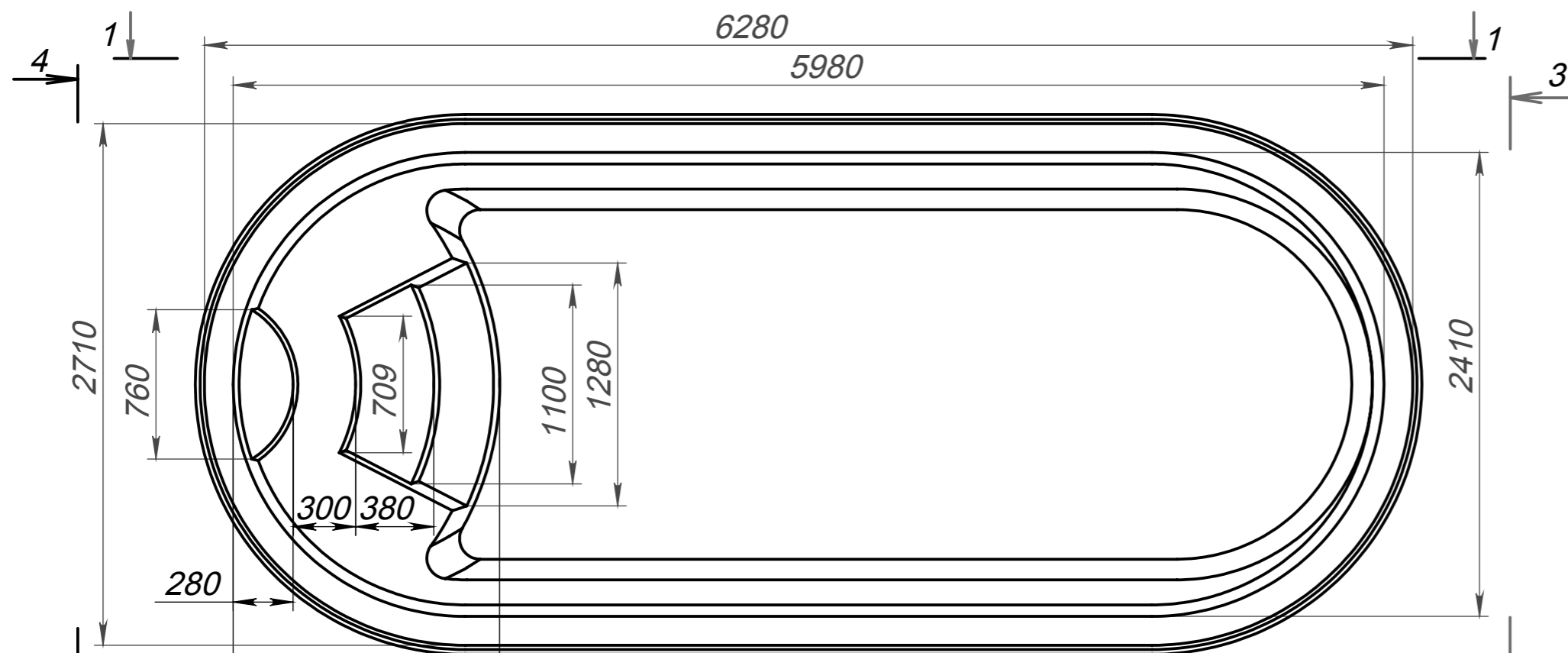
Вид 1-1
