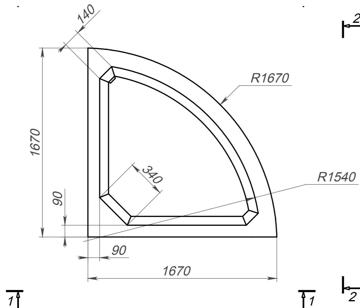
Вид 1-1
