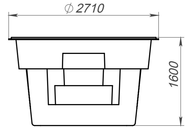
Вид 4-4
