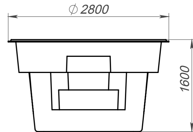
Вид 4-4
