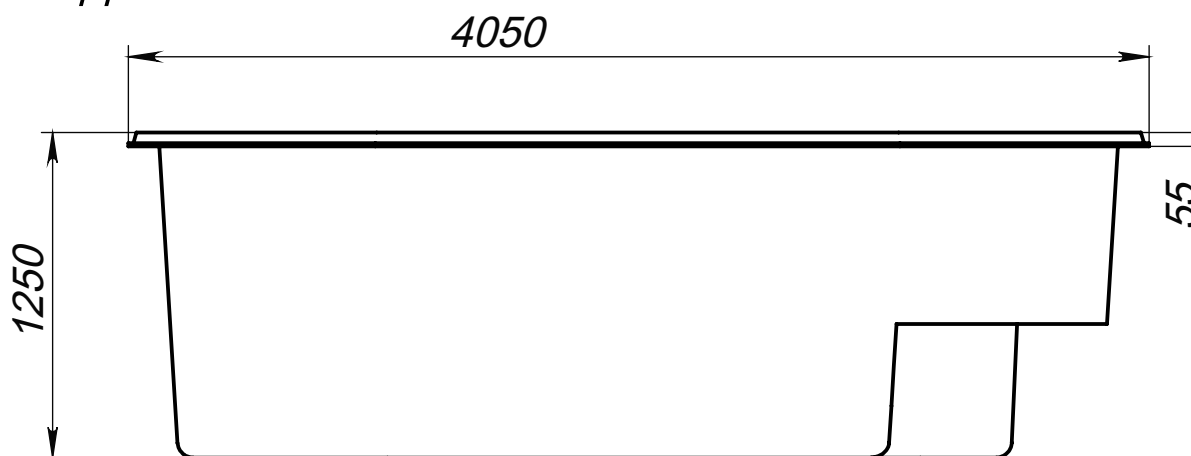
Вид 2-2
