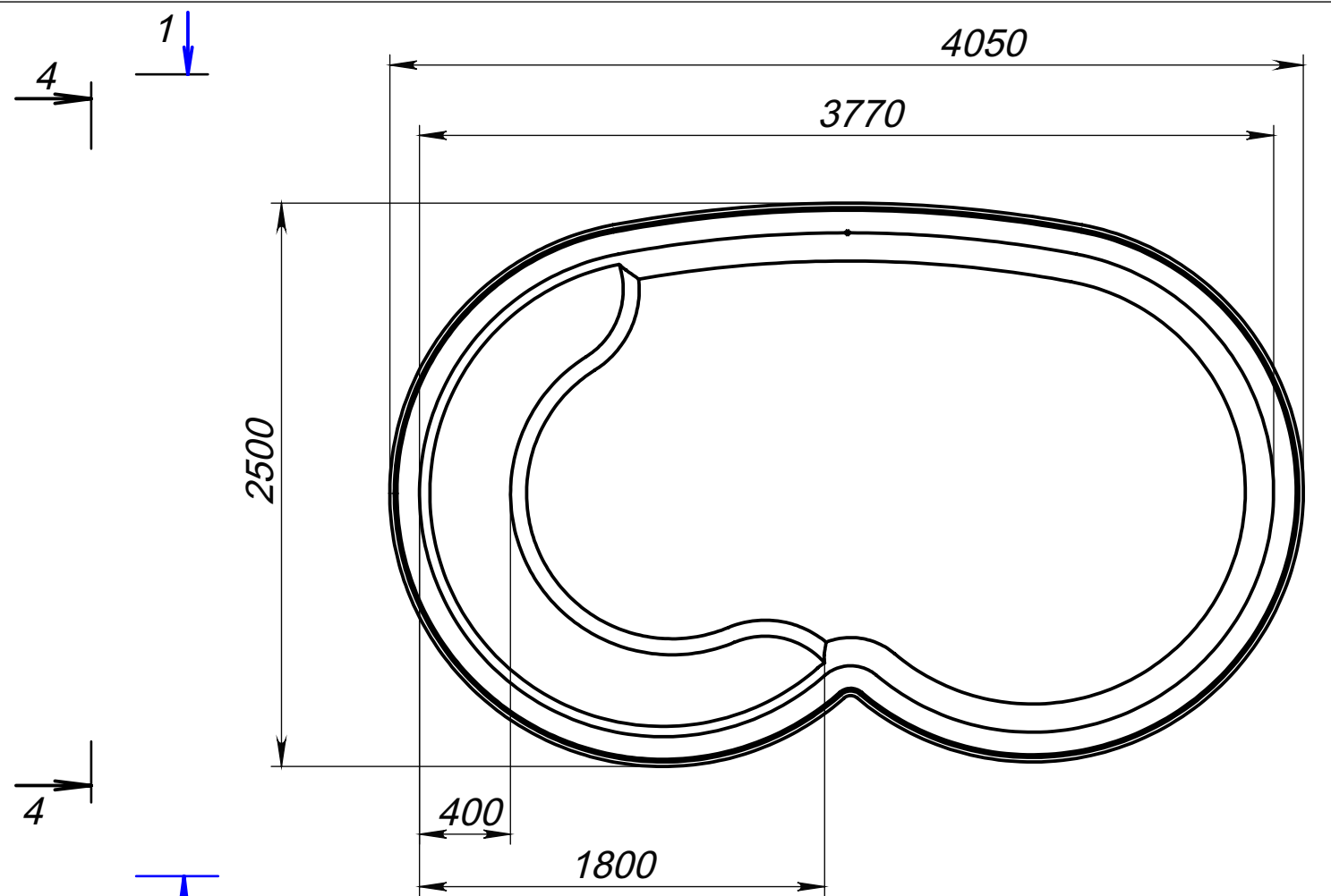
Вид 1-1
