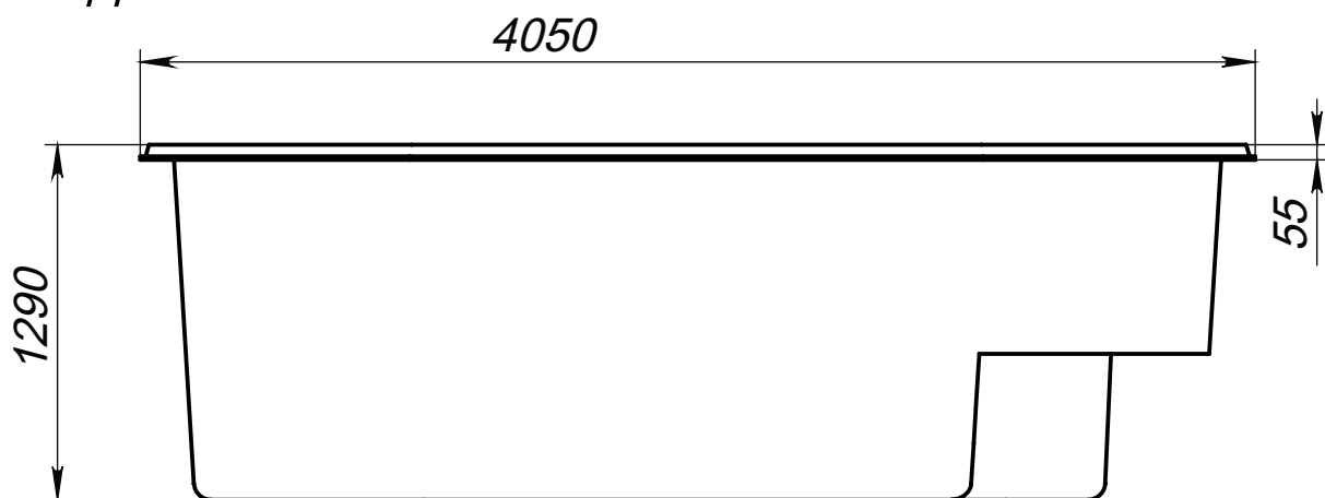
Вид 2-2
