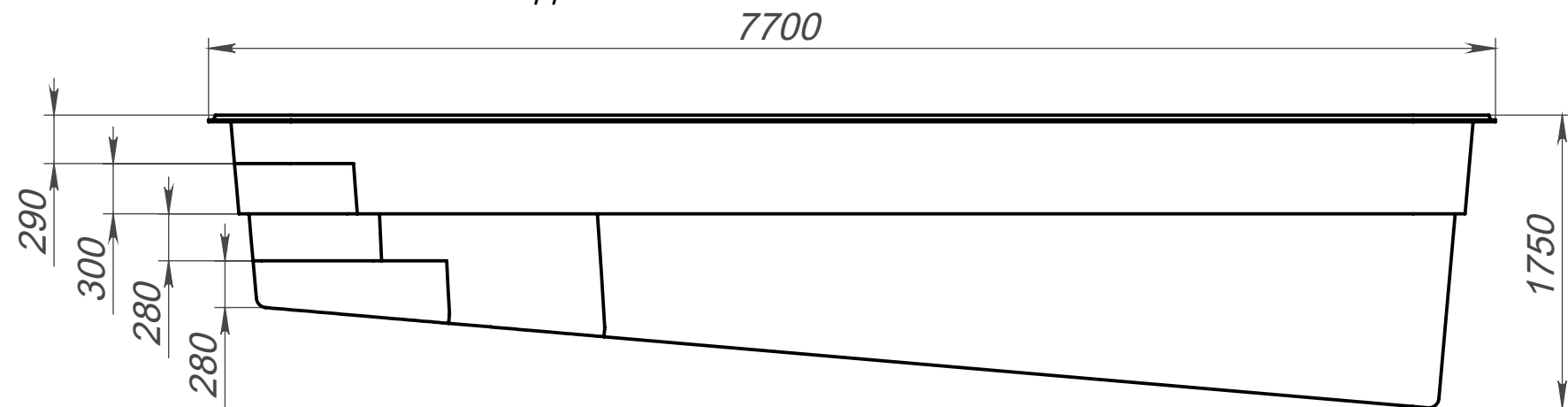
Вид 2-2
