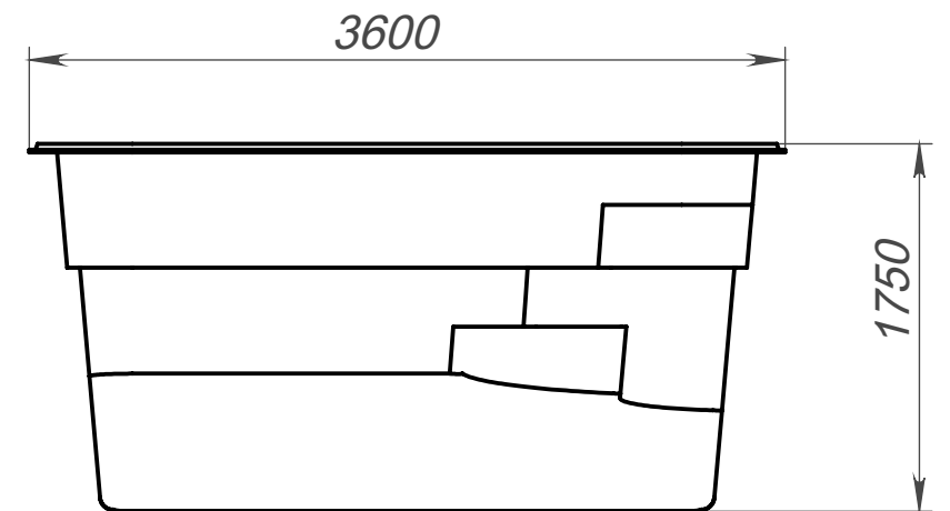
Вид 4-4
