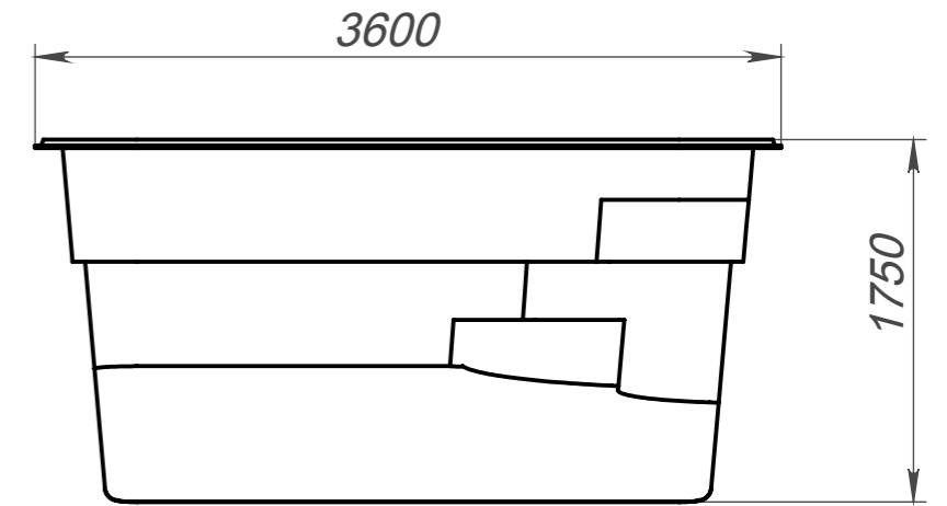
Вид 4-4
