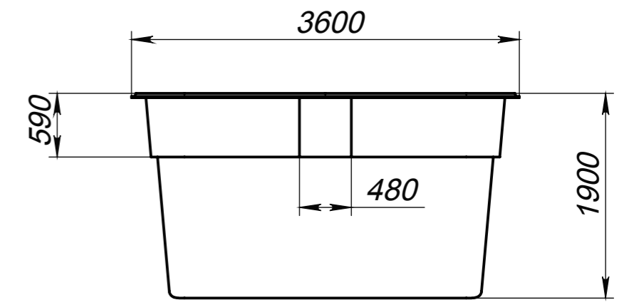
Вид 3-3
