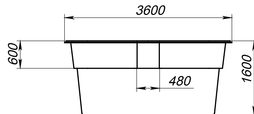
Вид 3-3
