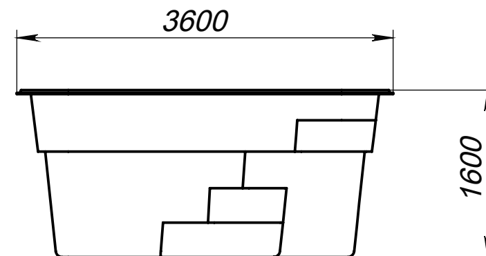
Вид 4-4
