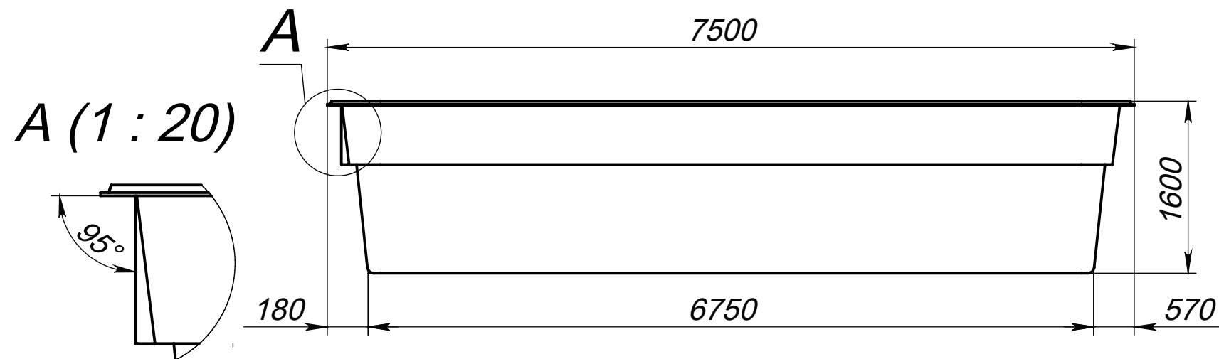
Вид 1-1
