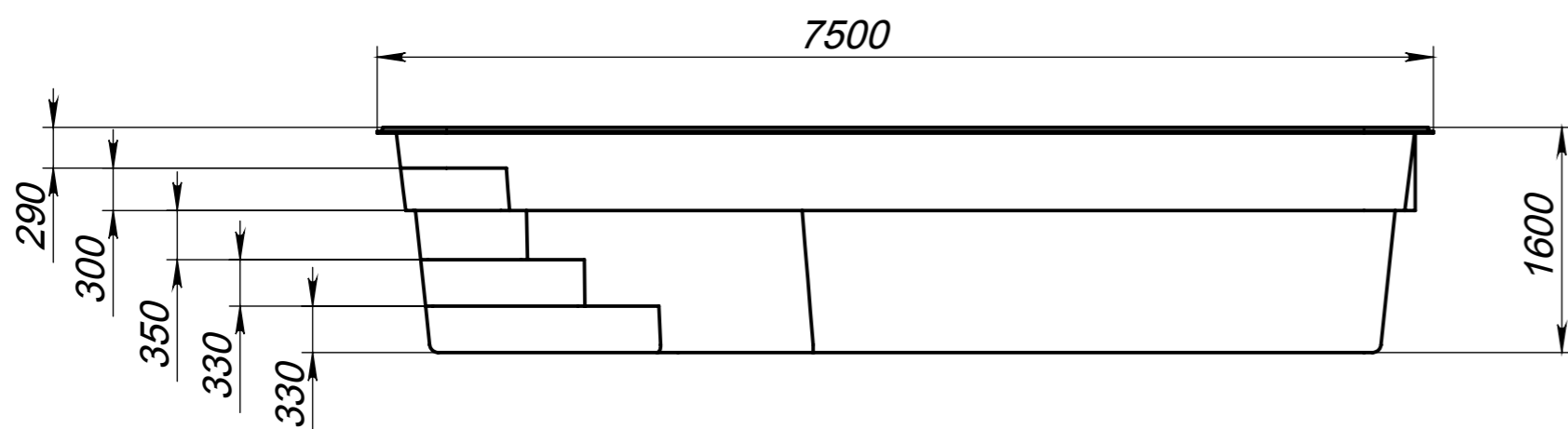
Вид 2-2
