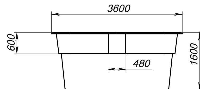
Вид 3-3
