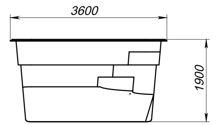
Вид 4-4
