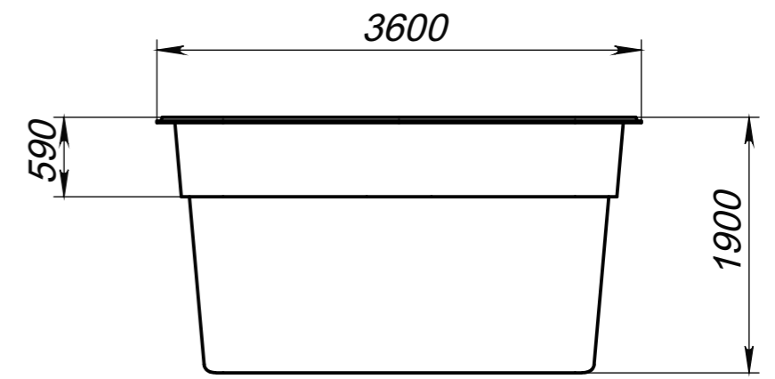
Вид 3-3
