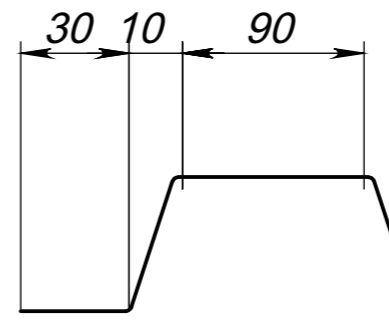
А (1 : 25)
